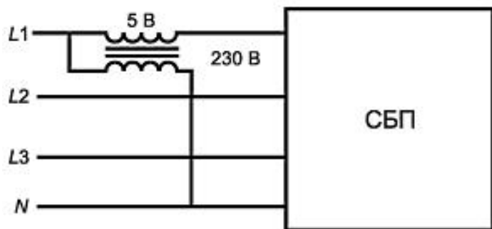
Рисунок D.1 - Амплитудная несимметрия
