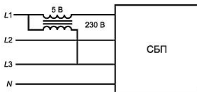
Рисунок D.2 - Фазовая несимметрия
